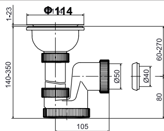
T-739 DN50/DN40 Sifon bez priključka, pileta Ø114 mm
