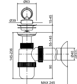
P-957 C DN40 Sifon za umivaonik metalna pileta
