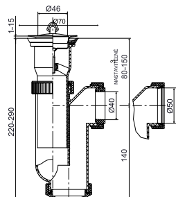
T-705 DN50/DN40 Sifon za sudoper bez preliva i priključka za perilicu
