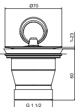
T-900C 5/4" Ispusni komplet-pileta 5/4"x63 met.
