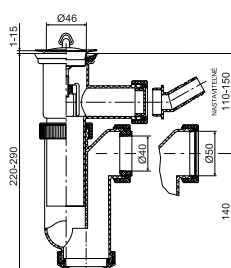
T-707 DN50/DN40 Sifon za sudoper bez preliva sa priključkom za perilicu
