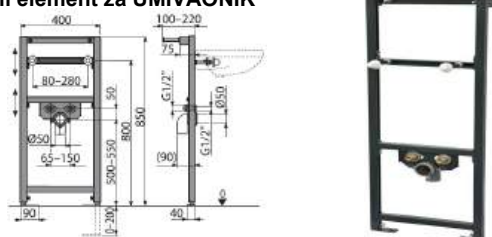
A104 Montažni element za UMIVAONIK
