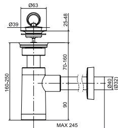
P-967CM DN40 Sifon za umivaonik -pileta metalna
