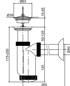
T-1015C DN40 Sifon za umivaonik metalna pileta
